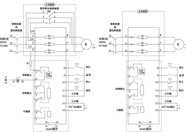
图5-1a 旁路型
