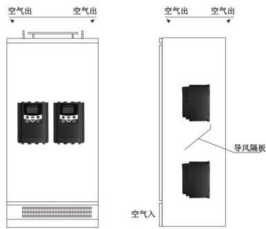
图3-2: 横向布局安装
