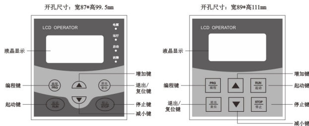
图7-1a 在线器显示操作面板
