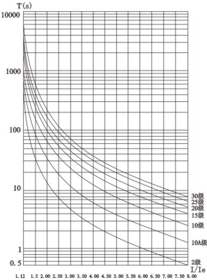
IEC60974-4-2电机热态保护曲线
