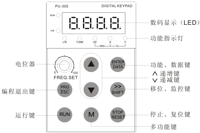
图 4-2 操作键盘布局图
