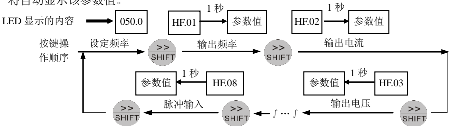
图 4-6 待机状态参数显示操作示例
