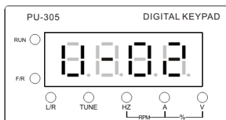
加速中过流 图 4-4 故障报警显示状态
