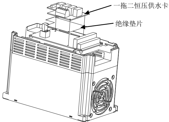
图 9-1 一拖二恒压供水卡安装示意图
