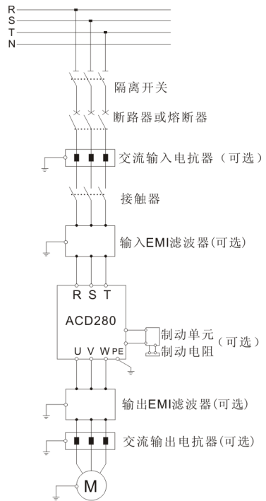
图 3-5 变频器与选配件的连接
