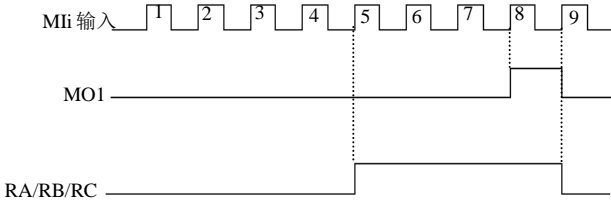
图 6-34 设定计数值给定和指定计数值给定示意图
