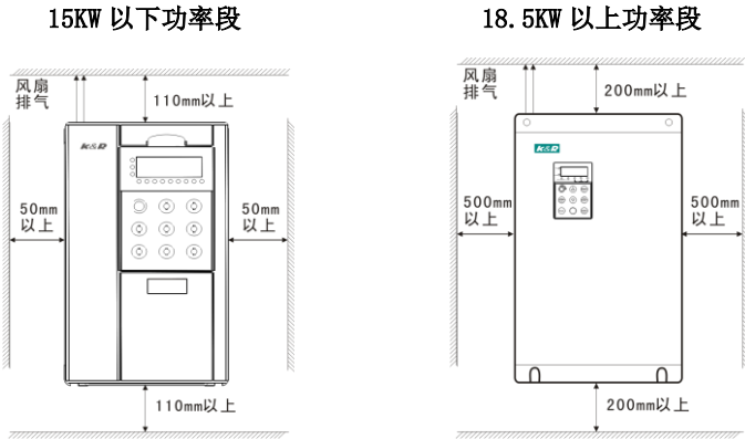
图 3-1 安装的间隔距离图
