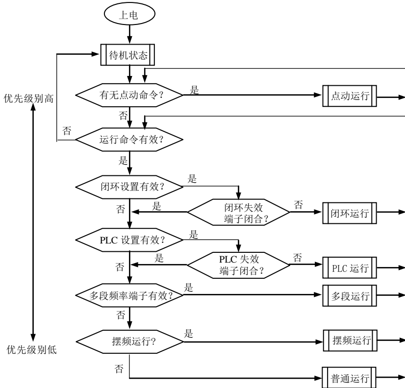
图 4-1 ACD280 变频器运行状态的逻辑程序
