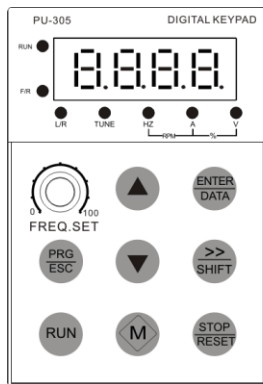
图 a 上电初始化， 显示 8.8.8.8。
