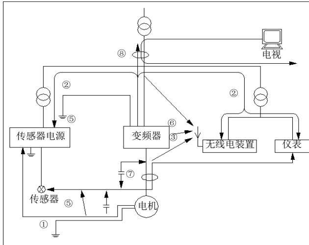
图 3-14 噪声干扰的传播路径示意图
