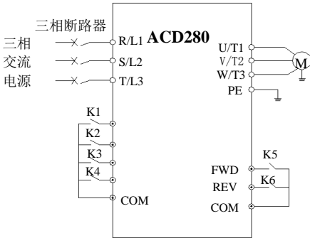
图 6-25 多段速运行接线图
