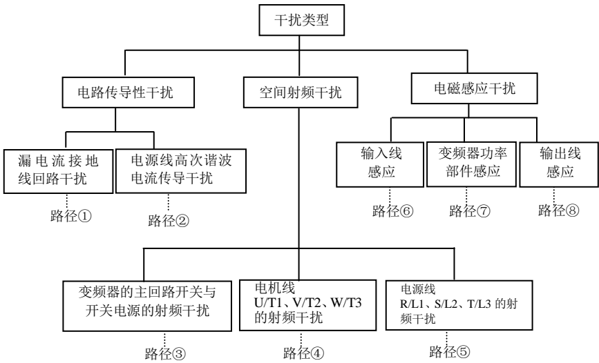
图 3-13 噪声干扰的分类
