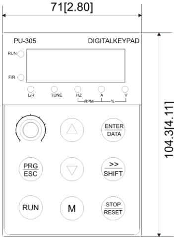
图 2-4 a 外形图
