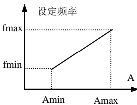
(1)正作用特性
