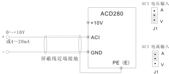
图 3-9 ACI 端子配线图
