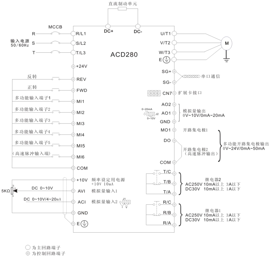
图 3-6 基本配线图
