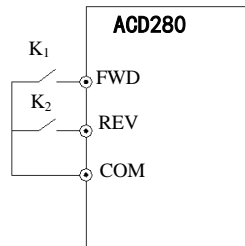
图 6-27 两线式运转模式 1
