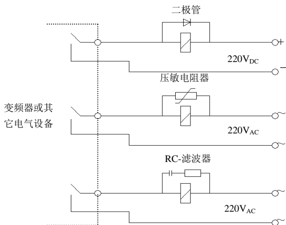
图 3-16 电磁开关类电器的安装要求
