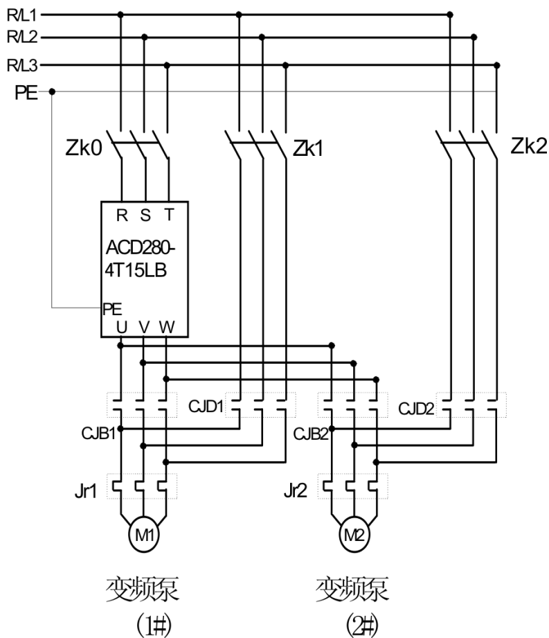
图 9-3 一次连线图
