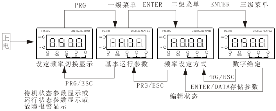
图 4-5 操作键盘显示状态的切换
