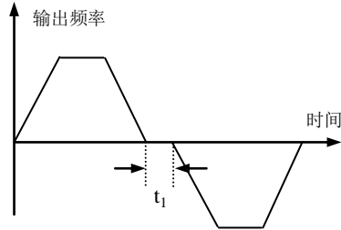
图 6-10 正反转死区时间
