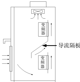
图 3-2 多台变频器的安装示意图
