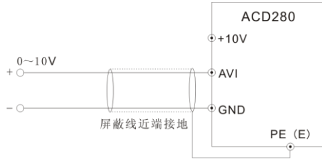
图 3-8 ACI 端子配线图
