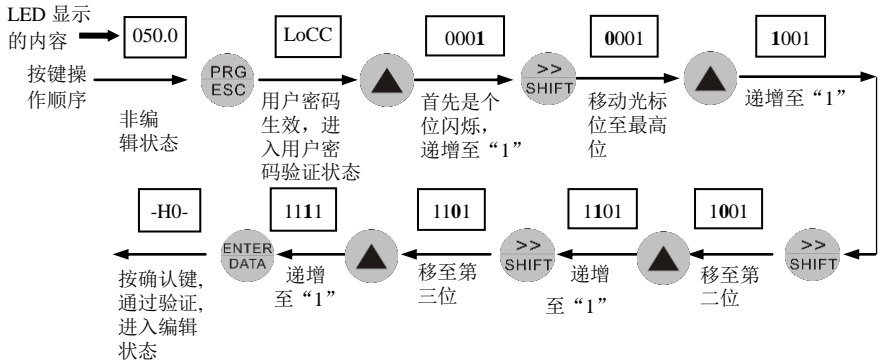
图 4-10 输入用户密码进入功能码操作的示例
