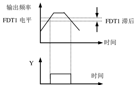
图 6-33 频率水平检测示意图
