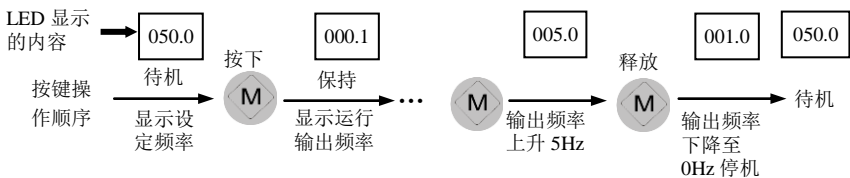
图 4-9 点动运行操作示例
