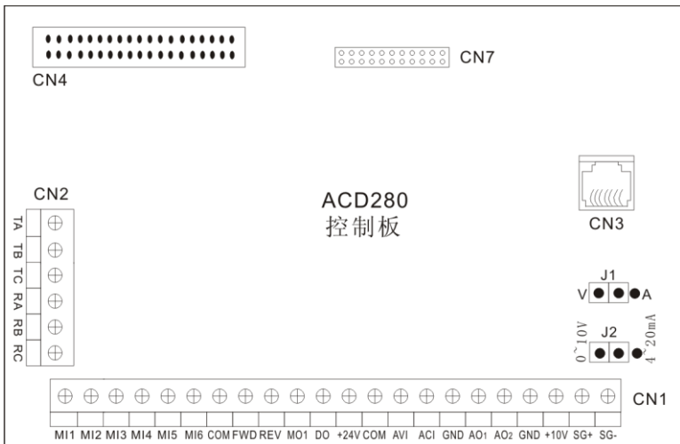
图 3-7 控制板的跳线开关位置示意图
