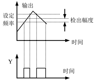
图 6-32 频率到达信号输出示意图
