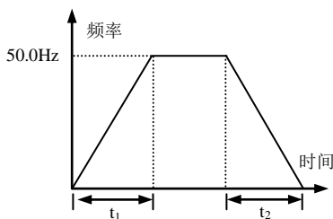
图 6-4 直线加减速
