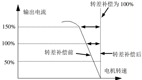
图 6-11 转差频率补偿示意图
