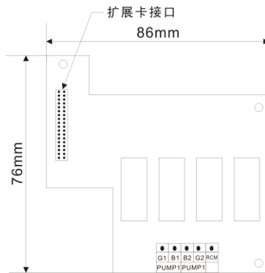
图 9-2 一拖二恒压供水卡外形尺寸示意图
