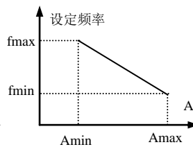
(2)反作用特性
