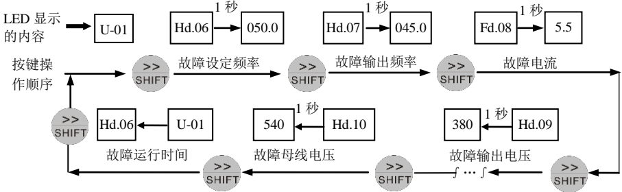
图 4-11 故障状态查询操作示例
