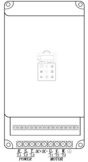
图 3-4 主回路简单配线
