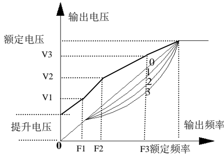
图 6-3 V/F 曲线
