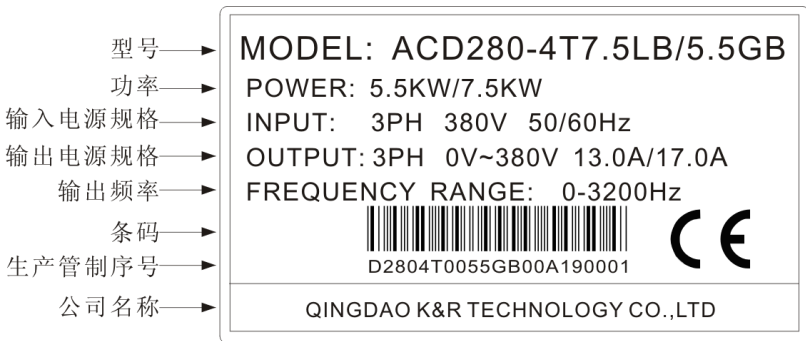
图 2-2 变频器铭牌
