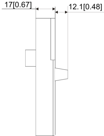
图 2-4 b 外形图
