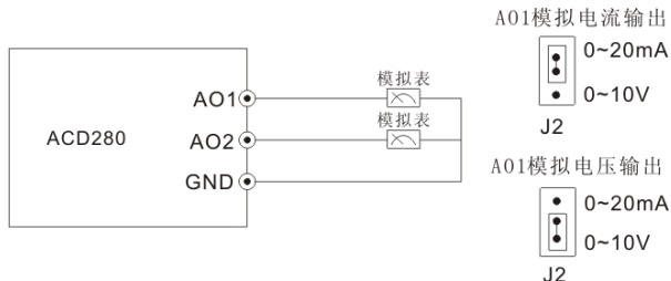
图 3-10 模拟输出端子配线图
