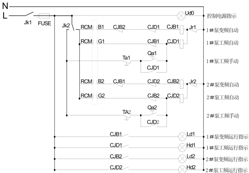
图 9-4 二次连线图
