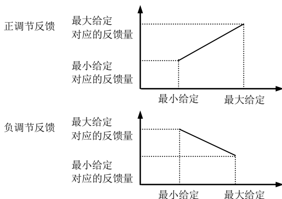
图 6-21 给定、反馈曲线示意图
