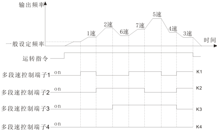
图 6-24 多段速运行示意图
