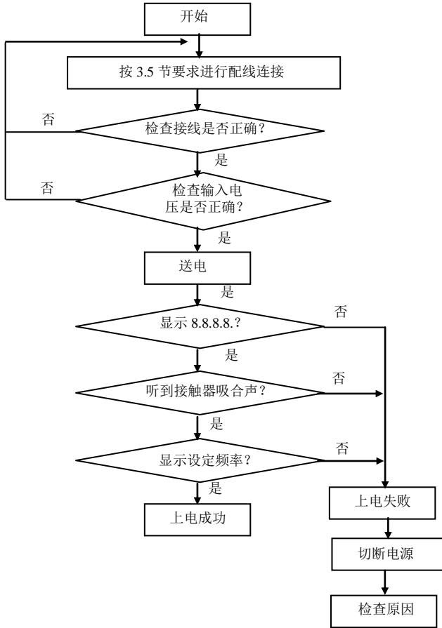
图 4-12 变频器初次上电操作流程
